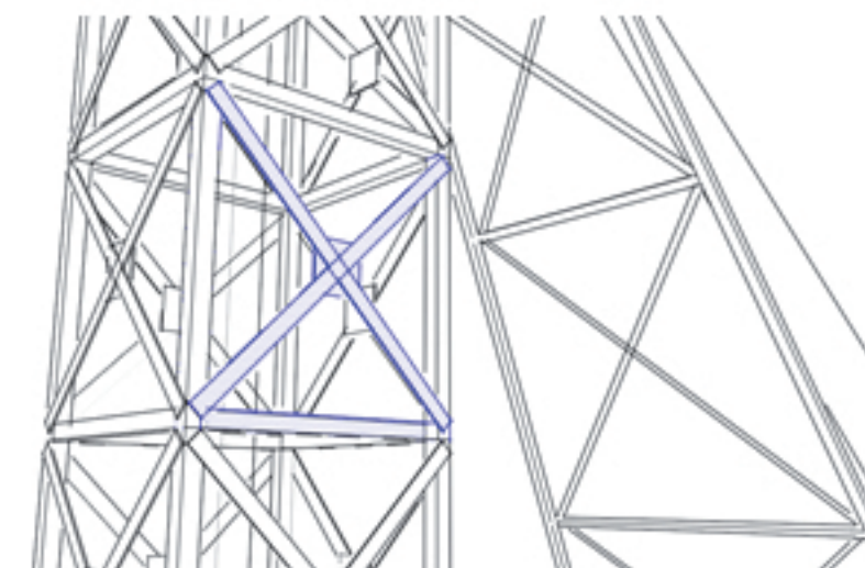
Stütze, Riegel, Verbände und Knotenblech
